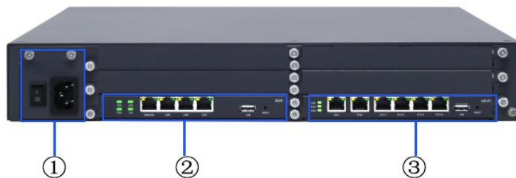
图 1-1 IAD100-4E1 前面板图
