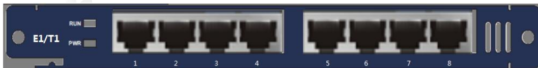
图 1-5 IAD100-8E1 8E1/T1 数字中继板外观图
