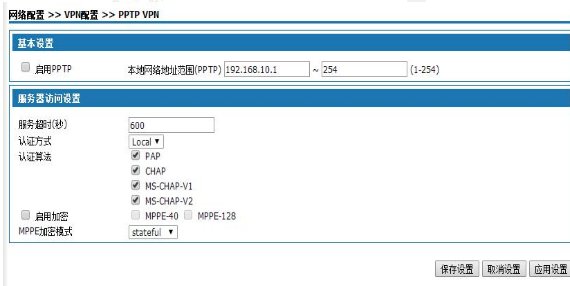
图 5-32 PPTP VPN-基本设置
