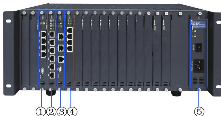
图 1-1 IAD100-8E1 前面板图
