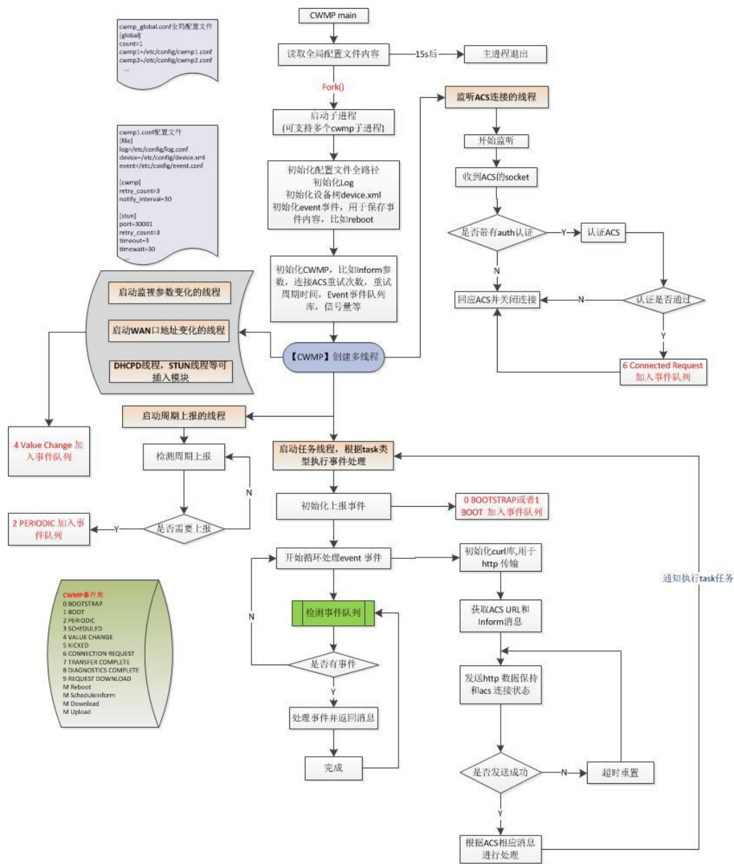
SIP-T800话机的TR069工作流程图：
